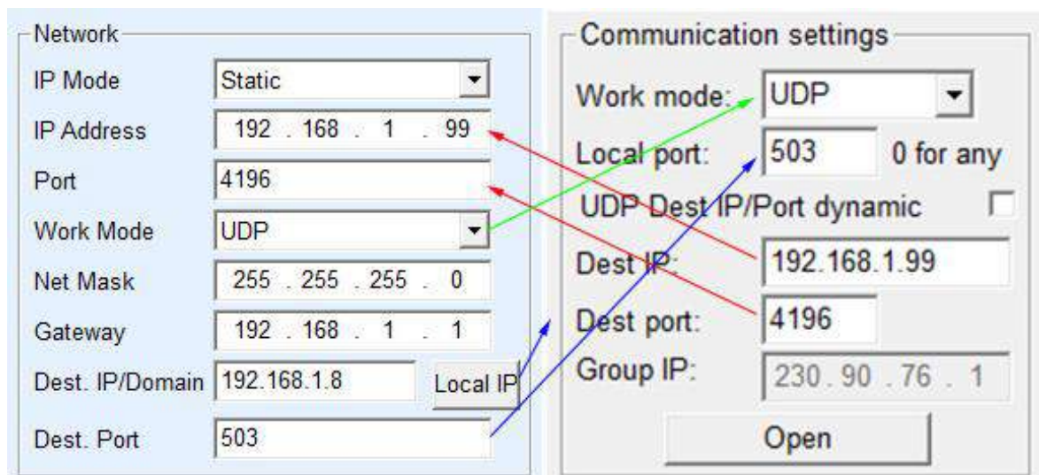
Figure 28 UDP mode Parameter Configuration
